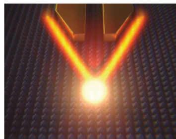
Focalizado de Nanoluz mediante el uso de nanoantenas de oro (www.scixel.es)
